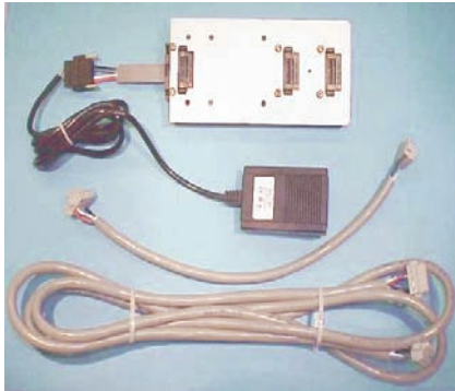
Mini network
