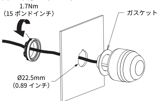
図3 - 取付け (パネル)
