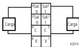
1734-OB2E
