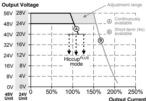
Fig. 1/ Bild 1 Output Characteristic /Ausgangskennlinie, typ.
