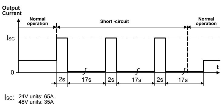
Fig. 2/ Bild 2 Hiccup PLUS Overload and Short-Circuit Behavior / Hiccup PLUS Überlast- und Kurzschlussverhalten, typ.
