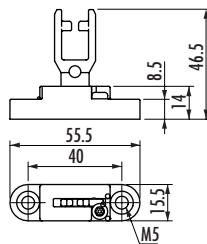
SEMI FLEXIBLE ACTUATOR
