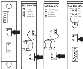
1747-AIC SLC 5/01 SLC 5/02 SLC 5/03
